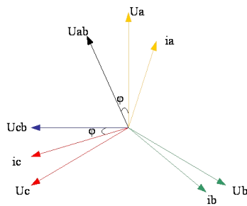
三相交流电相量图
