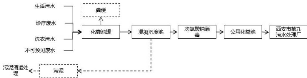
图 4-1 污水处理装置工艺流程图
