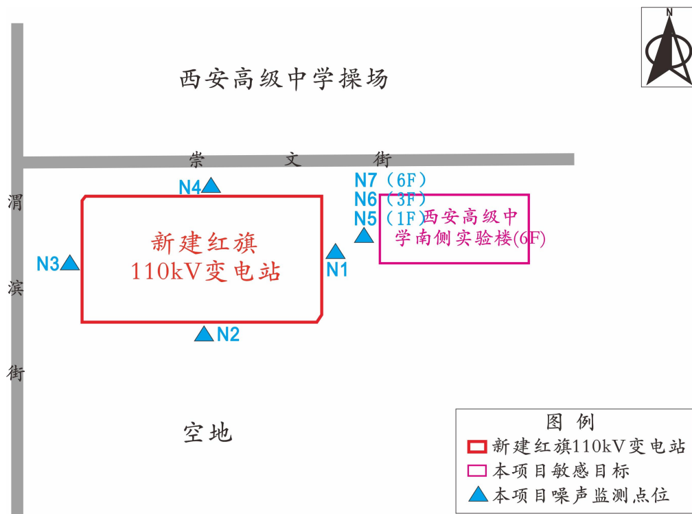
图 3-6 本项目新建西安红旗 110kV 变电站周围声环境监测点位示意图
