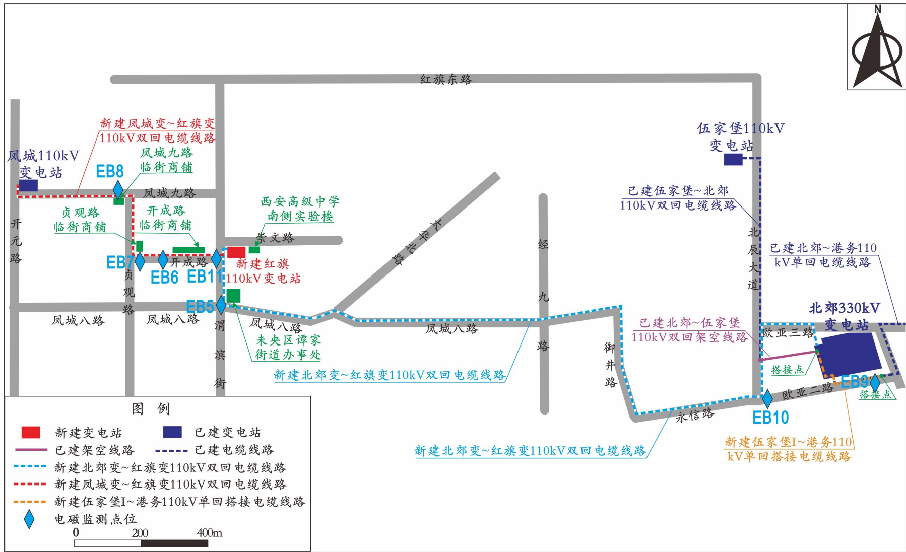
图 2 电缆线路及环境敏感目标电磁环境监测点位示意图
