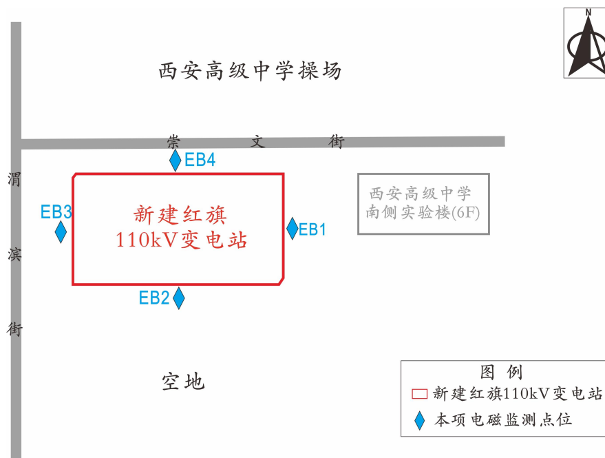
图 1 西安红旗 110kV 变电站电磁环境监测点位示意图
