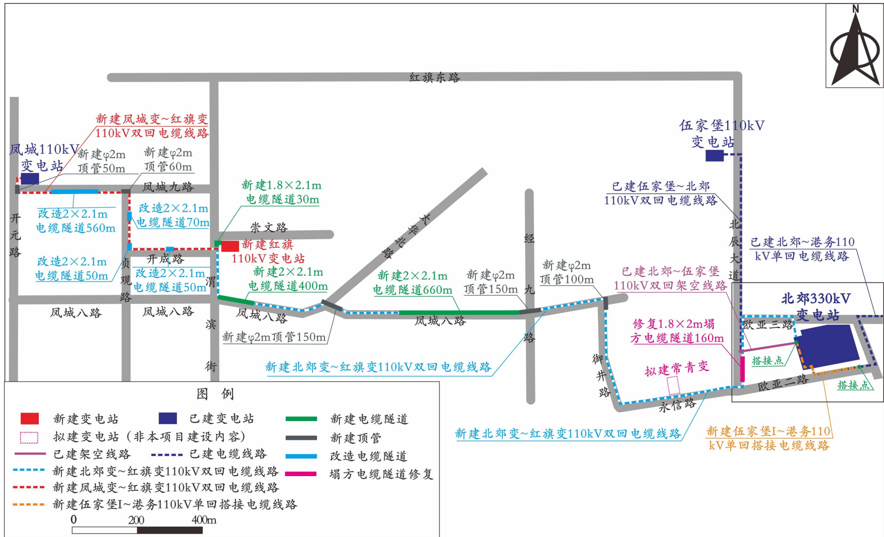
图2-2 本项目线路路径示意图
