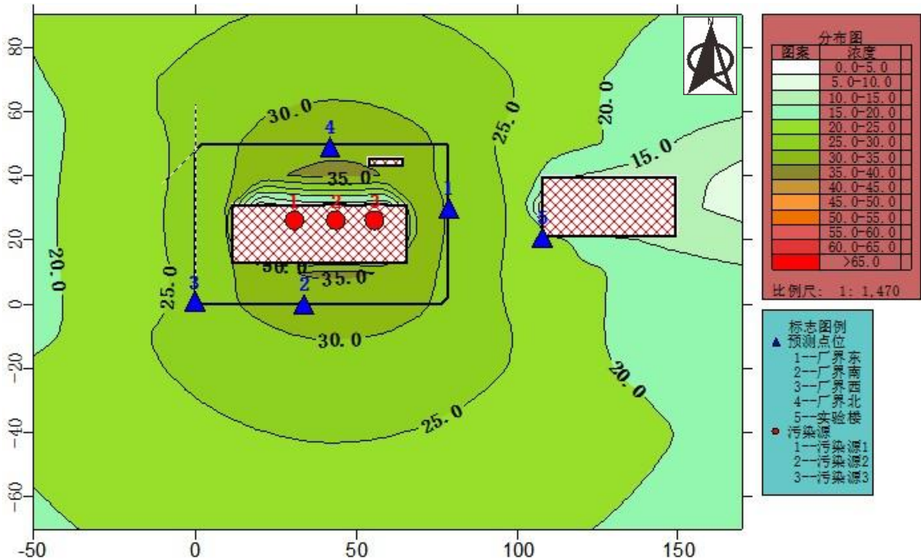
图 4-6 西安红旗 110kV 变电站等效噪声级预测图（西安高级中学南侧实验楼 3 层/7.5m）
