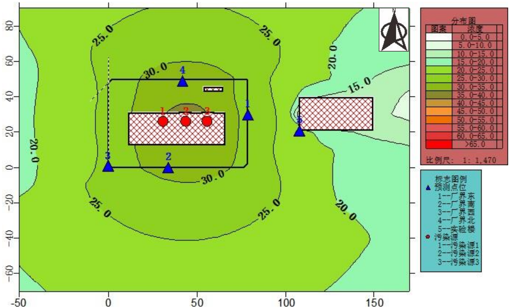
图 4-7 西安红旗 110kV 变电站等效噪声级预测图（西安高级中学南侧实验楼 6 层/16.5m）
