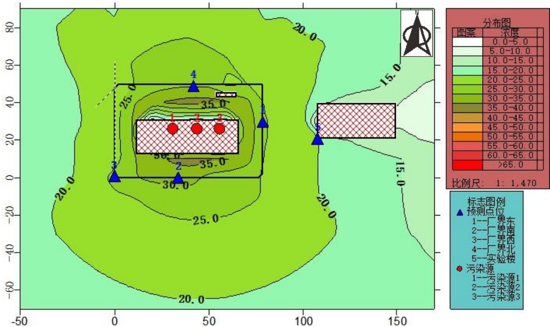
图 4-5 西安红旗 110kV 变电站等效噪声级预测图 (西安高级中学南侧实验楼 1 层/1.5m)
