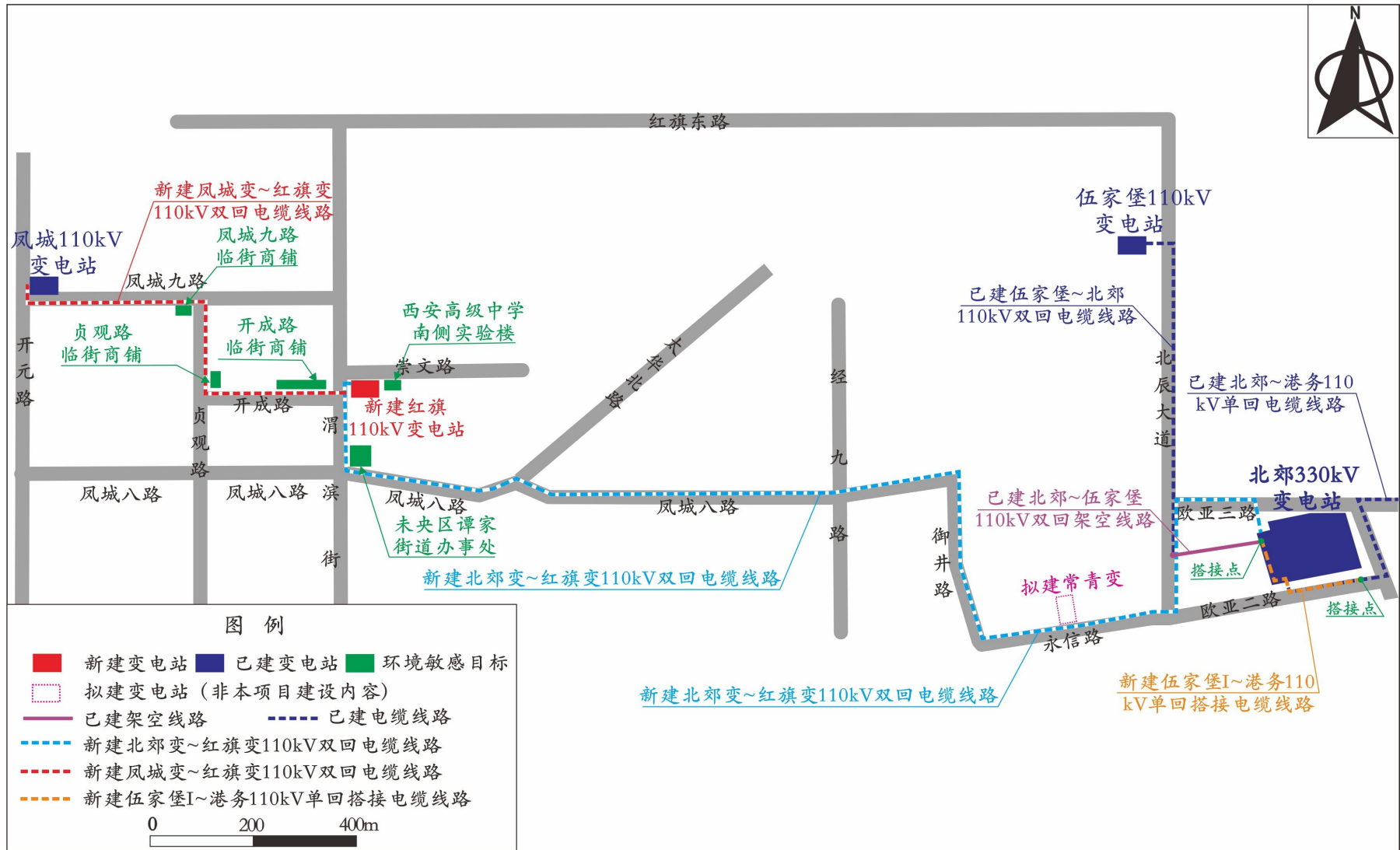
图 3-8 环境敏感目标分布示意图
