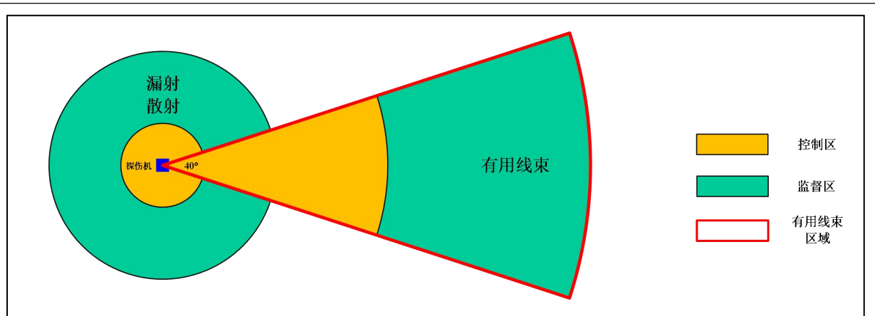
图 10-1 X 射线现场探伤时控制区和监督区划分示意图（定向探伤机）
