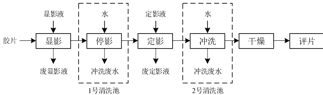
图 9-6 洗片工艺流程图
