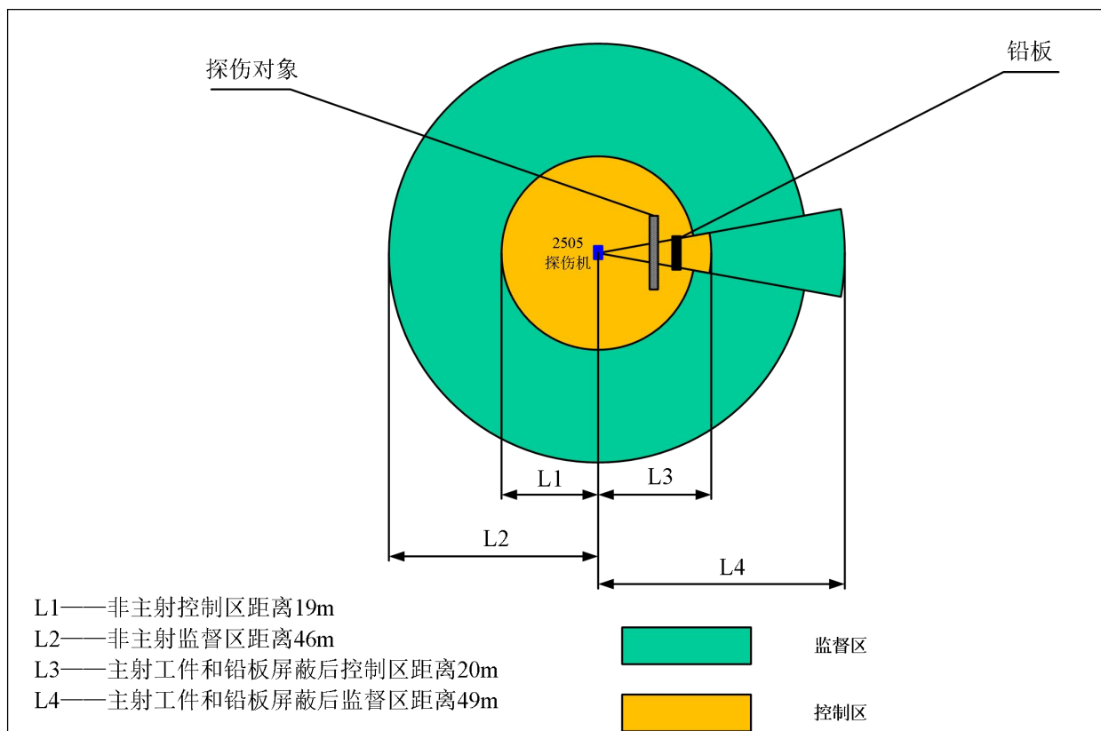
图 11-2 2505 型定向 X 射线探伤机控制区和监督区范围分区示意图(工件厚度 38mm+2mm 铅板)
