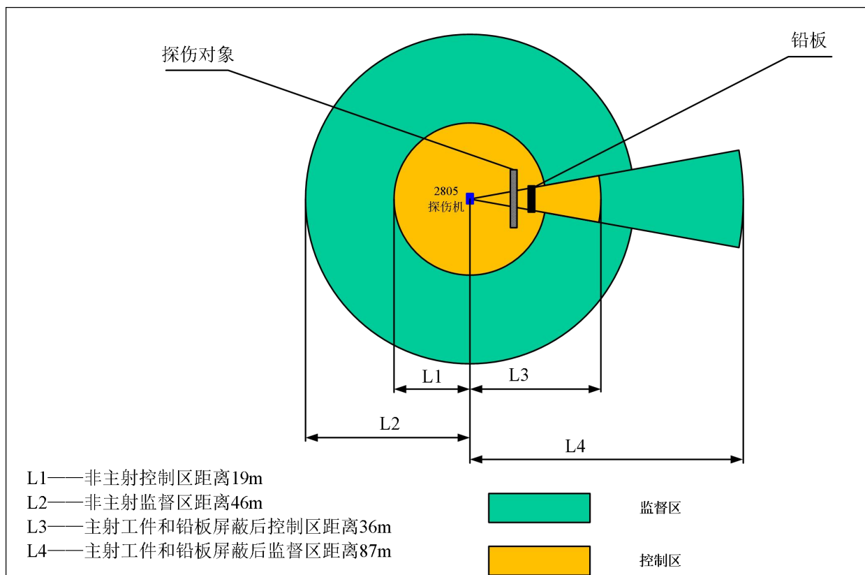
图 11-4 2805 型定向 X 射线探伤机控制区和监督区范围分区示意图(工件厚度 40mm+2mm 铅板)
