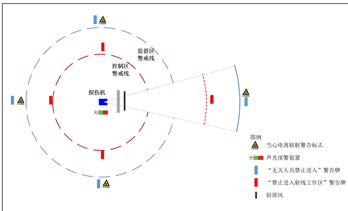
图 10-2 移动探伤现场辐射安全设施布置示意图
