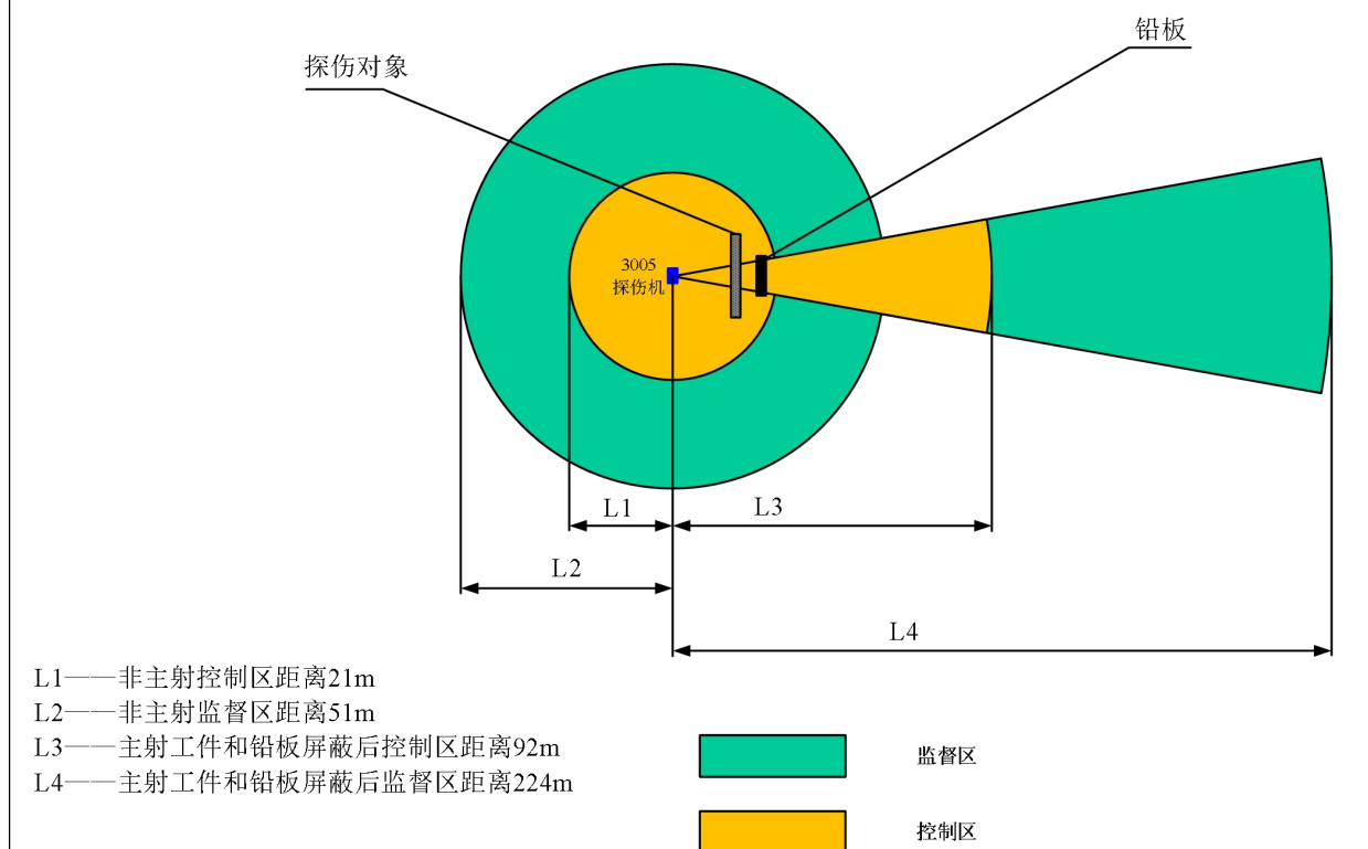
图 11-5 3005 型定向 X 射线探伤机控制区和监督区范围分区示意图(工件厚度 30mm+2mm 铅板)
