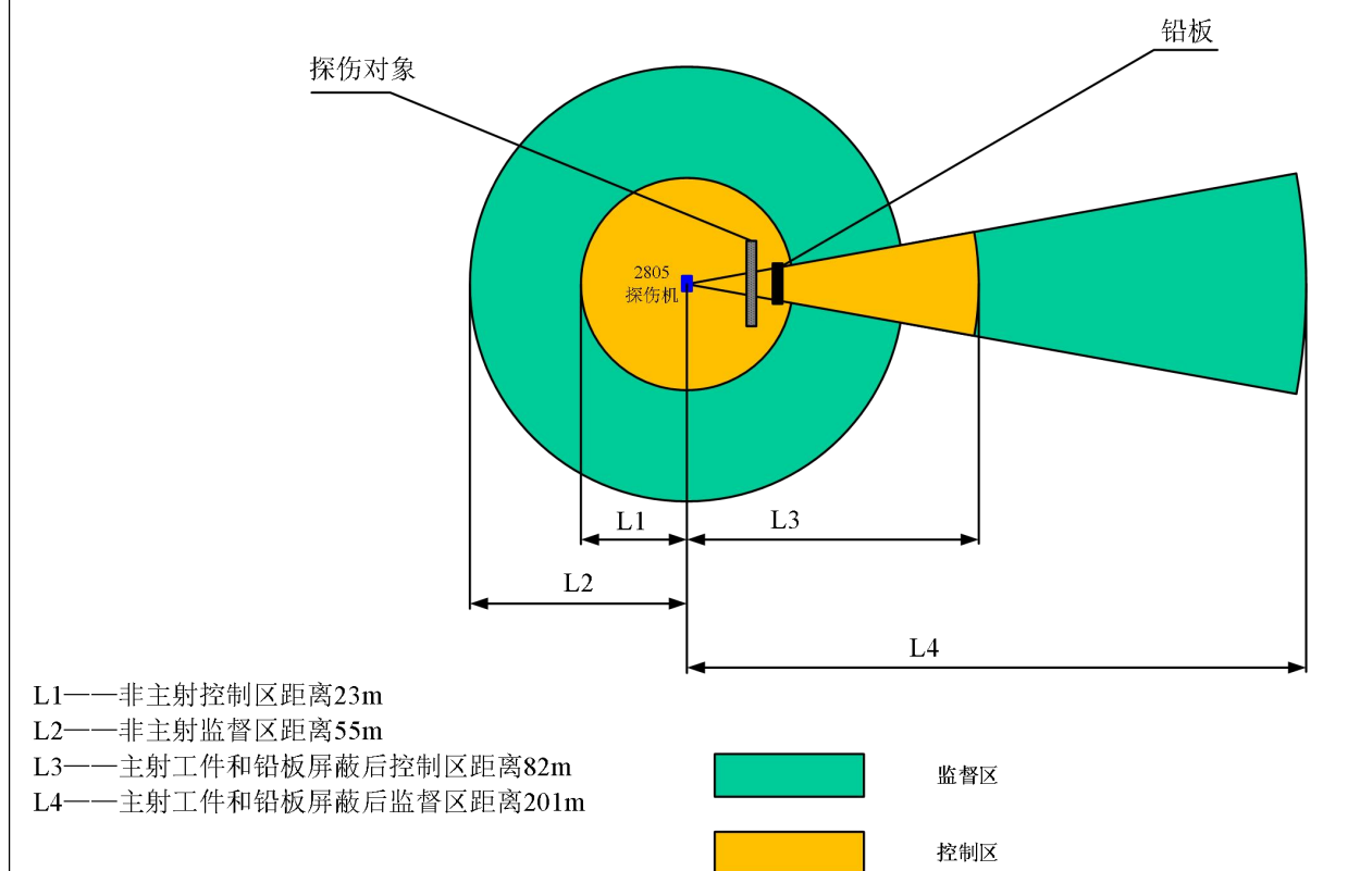
图 11-3 2805 型定向 X 射线探伤机控制区和监督区范围分区示意图(工件厚度 26mm+2mm 铅板)
