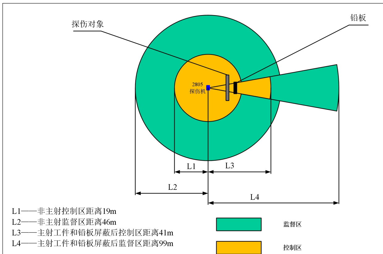
图 11-6 3005 型定向 X 射线探伤机控制区和监督区范围分区示意图(工件厚度 45mm+2mm 铅板)
