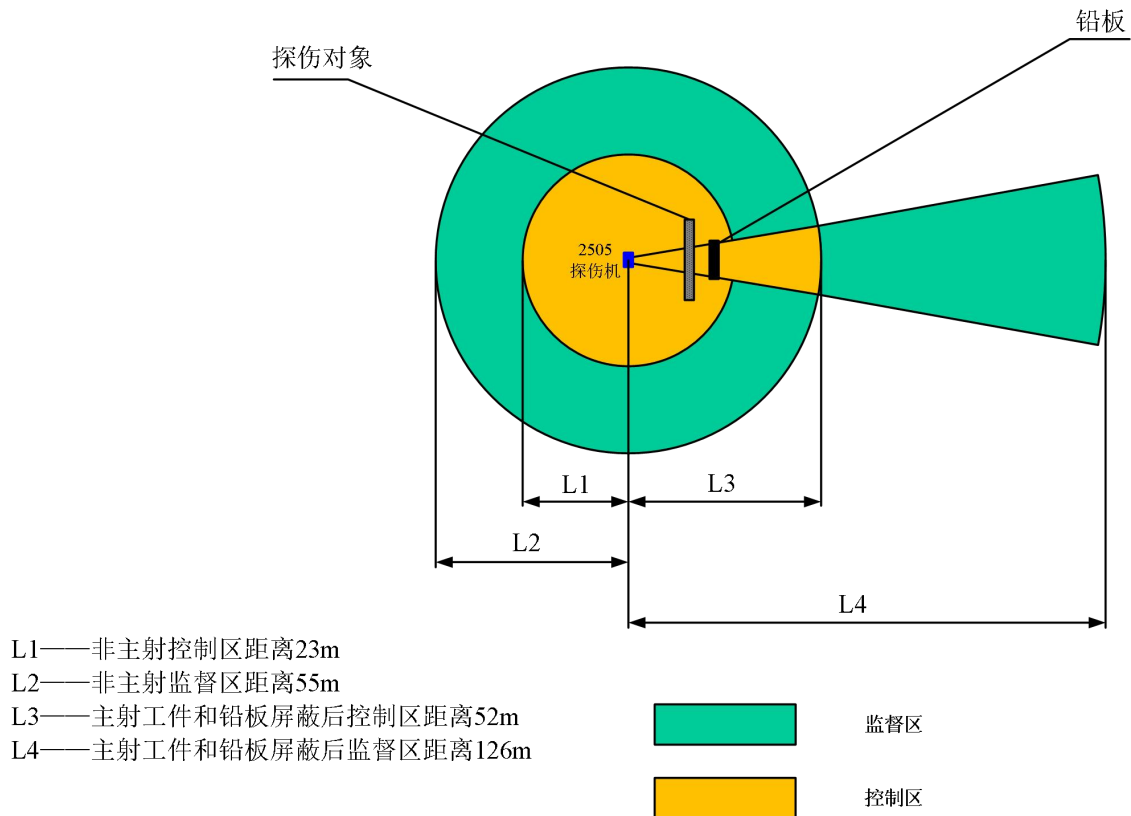
图 11-1 2505 型定向 X 射线探伤机控制区和监督区范围分区示意图(工件厚度 24mm+2mm 铅板)
