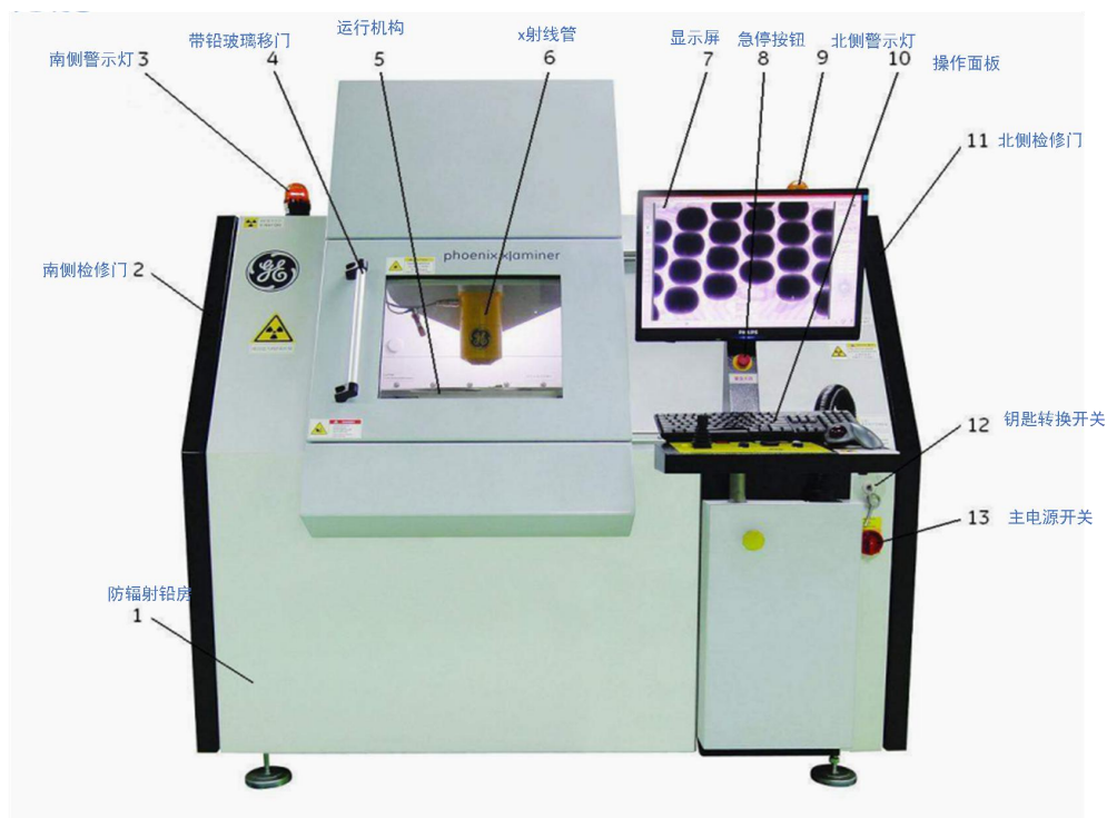
图 9-3 phoenix x|aminer 高功率 X 射线检测系统结构示意图
