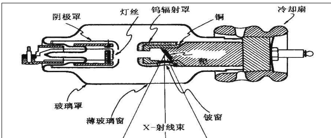
图 9-2 X 射线管的结构
