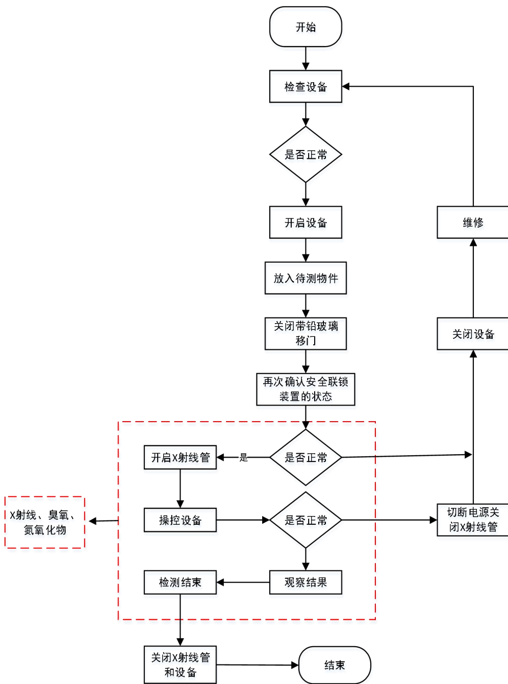
图 9-4 phoenix x|aminer 高功率 X 射线检测系统工作流程及产污环节图
