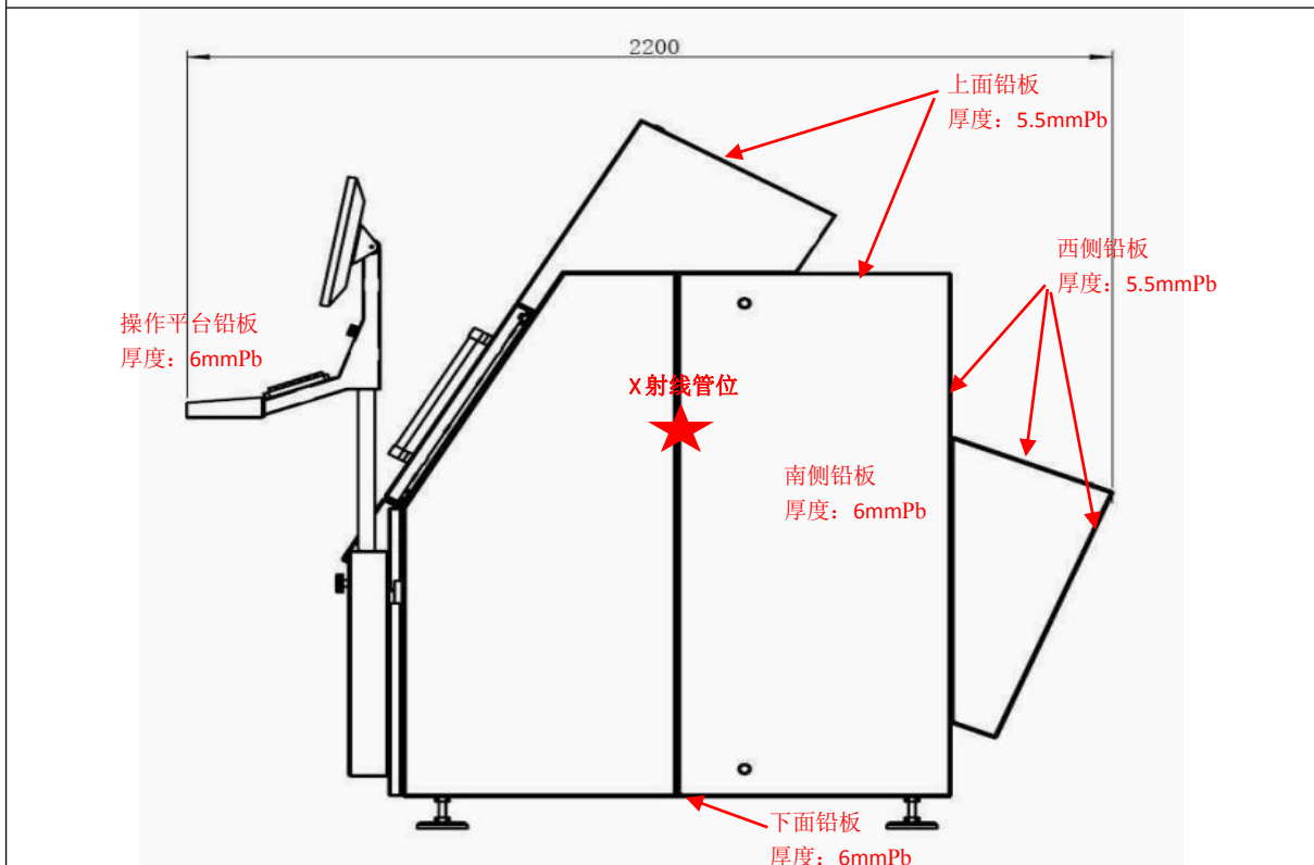
侧视图
