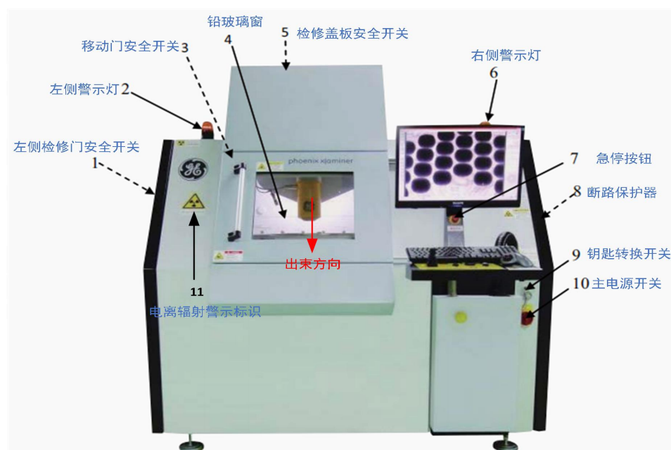
图 10-2 phoenix x|aminer 高功率 X 射线检测系统防护设施示意图
