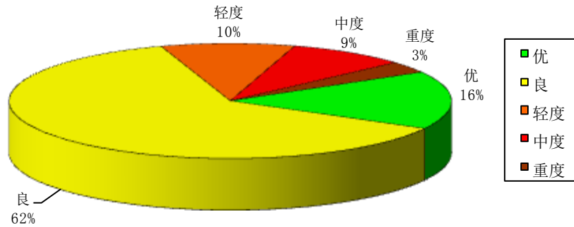
1 2023 年四季度环境空气质量分级比例
