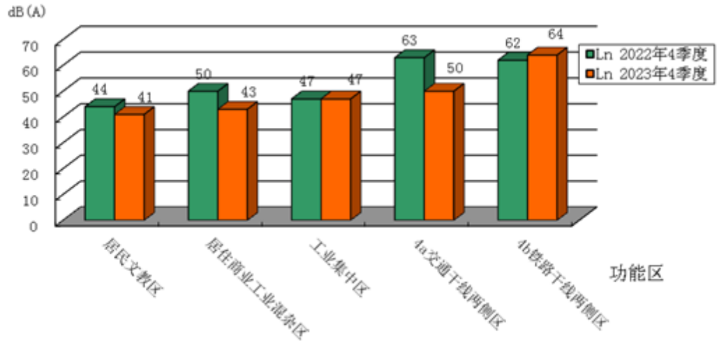
图 13 2023 年四季度夜间噪声与上年同期变化比较
