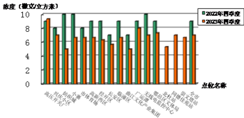
图3 2023年四季度国控点二氧化硫季均值与上年同期比较
