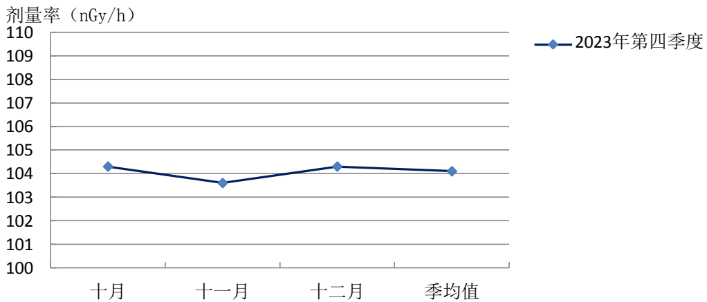
图 14 2023 年第四季度辐射自动检测值变化曲线图
