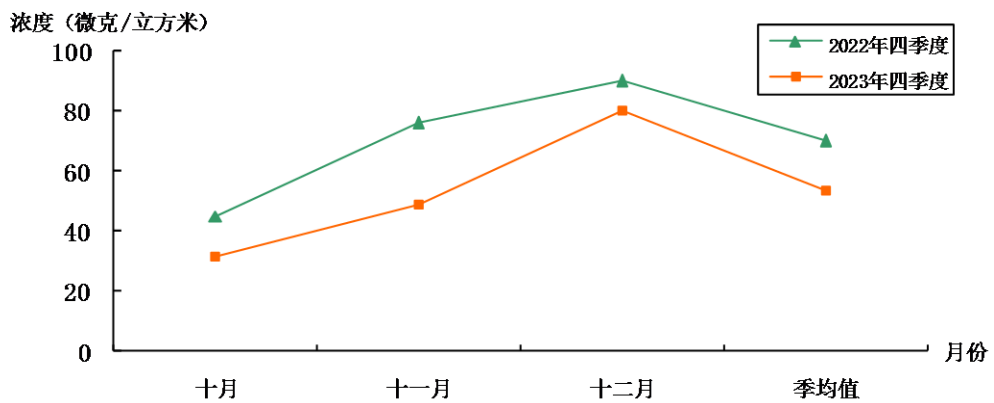
图10 2023年四季度全市颗粒物PM 2.5 月均值与上年同期比较
