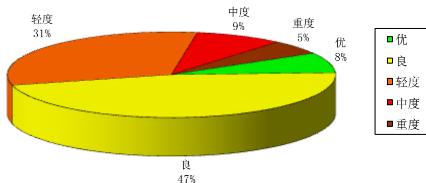
图 2 2022 年四季度环境空气质量分级比例
