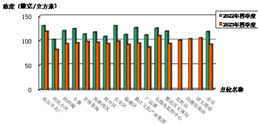
图7 2023年四季度国控点颗粒物PM 10 季均值与上年同期比较
