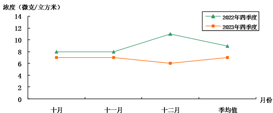
图4 2023年四季度全市二氧化硫月均值与上年同期比较
