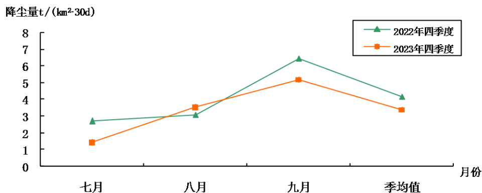
图 11 2023 年四季度降尘量与上年同期比较
