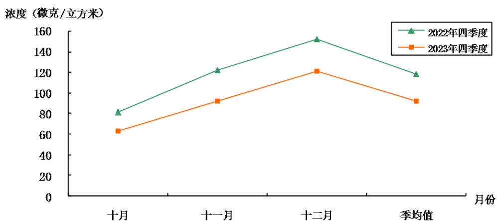
图8 2023年四季度全市颗粒物PM 10 月均值与上年同期比较
