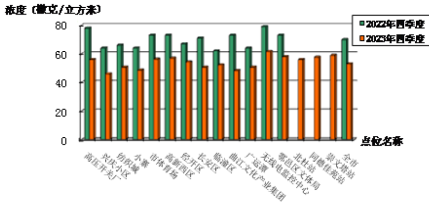
图9 2023年四季度国控点颗粒物PM 2.5 季均值与上年同期比较
