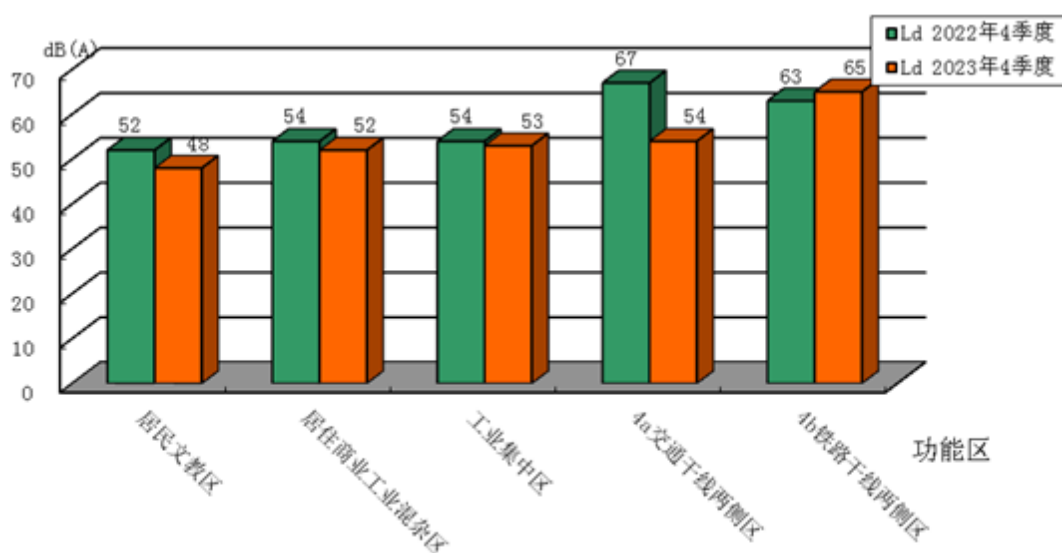
图 12 2023 年四季度昼间噪声与上年同期变化比较
