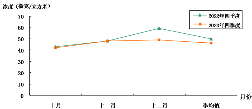
图6 2023年四季度全市二氧化氮月均值与上年同期比较
