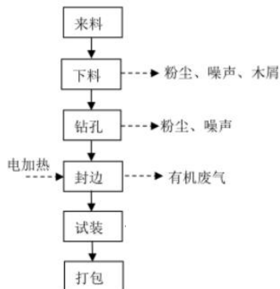
图 2 营运期工艺流程图
