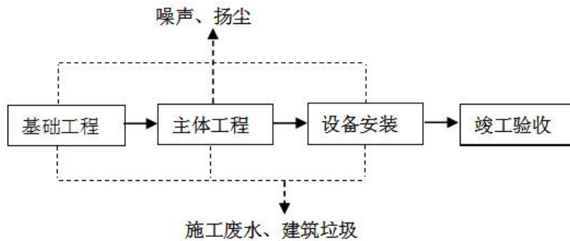
图 2 施工期工艺流程图
