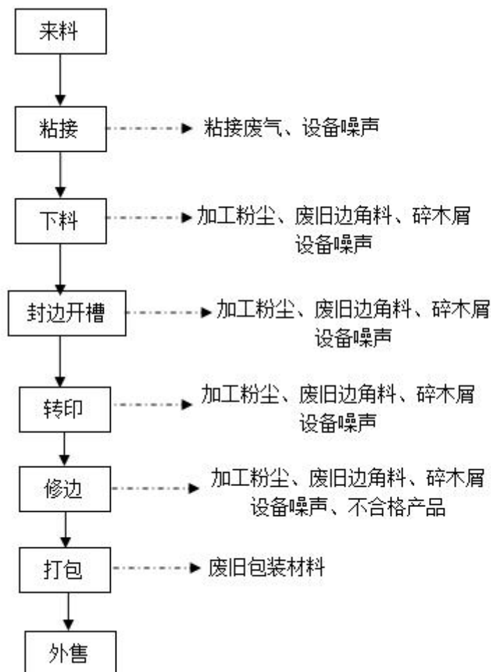
图2 营运期工艺流程图
